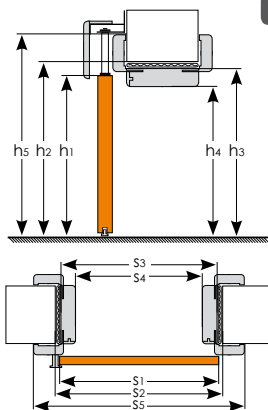
WYMIARY SKRZYDŁA I OBUDOWY MURU DO SYSTEMU NAŚCIENNEGO (mm):
