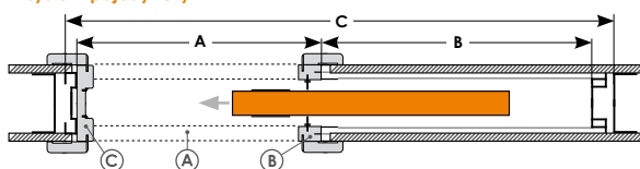
WYMIARY SKRZYDŁA I KASETY DO SYSTEMU CHOWANEGO W ŚCIANĘ (mm):
