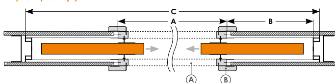
WYMIARY SKRZYDŁA I KASETY DO SYSTEMU CHOWANEGO W ŚCIANĘ (mm):
