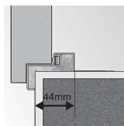
ościeżnica kątowa mała
