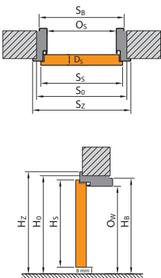
OŚCIEŻNICA METALOWA
