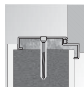
OPAL Montaż na dyble.
