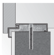
ościeżnica kątowa duża montaż na dyble
