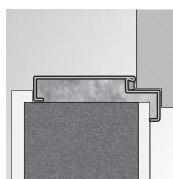
AGAT montaż bez dodatkowych elementów kotwiących
