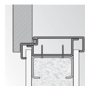
ościeżnica kątowa duża montaż na ścianie kartonowo-gipsowej
