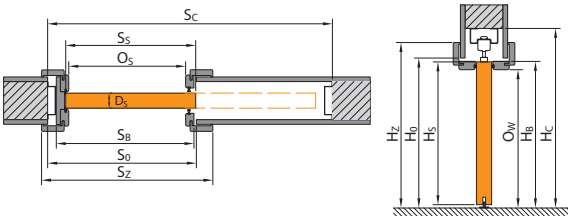
SYSTEM PRZESUWNY KOMPAKT
