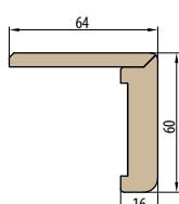
Kątownik z przedłużonym piórem do ościeżnicy regulowanej
