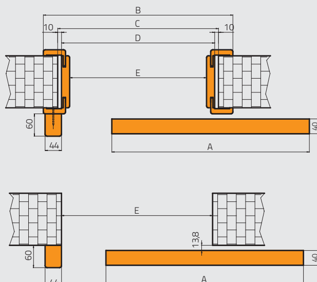
Rys. 2 Przekrój poziomy systemu przesuwnego ściennego - belka odbojowa prawa
