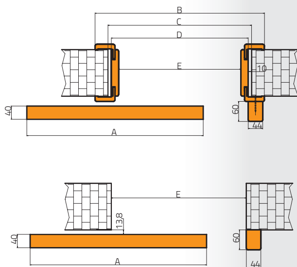
Rys. 1 Przekrój poziomy systemu przesuwnego ściennego - belka odbojowa lewa
