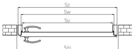
WYMIARY OŚCIEŻNIC STAŁYCH MU/U DO DRZWI DWUSKRZYDŁOWYCH W TECHNOLOGII STANDARD
